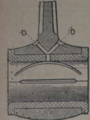
Figura 182.—Cabeza de biela. D: agujeros de engrase.
