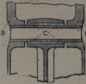
Figura 187.—Engrase del pie de biela. A: orificio superior, B: orificio inferior.
