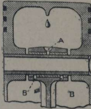
Figura 188.—Engrase del pie de biela por el aceite de cilindro. B: rebajo de retención del aceite, C: agujeros de engrase.
