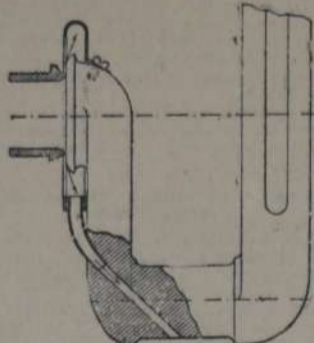
Figura 185.—Marcha del aceite en el engrase centrífugo de las cabezas de biela.
